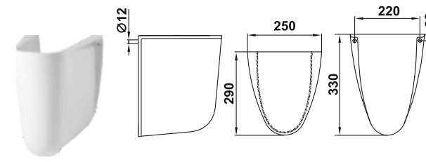
Пьедестал консольный Люкс Wall-hang column Lux
