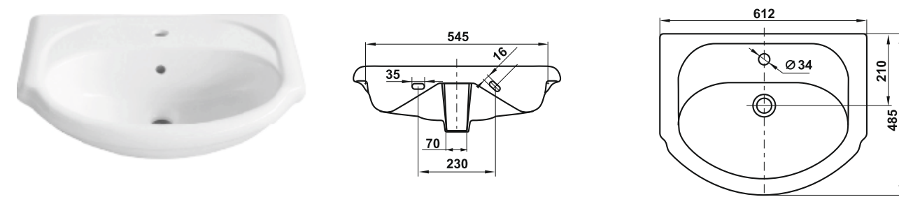
Умывальник мебельный Верона 61 Semi-recessed wash-basin Verona 61
